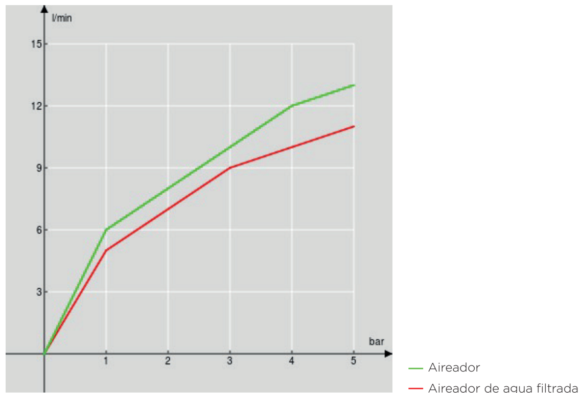
DIAGRAMA DE FLUJO: AGUA CALIENTE/FRIA
