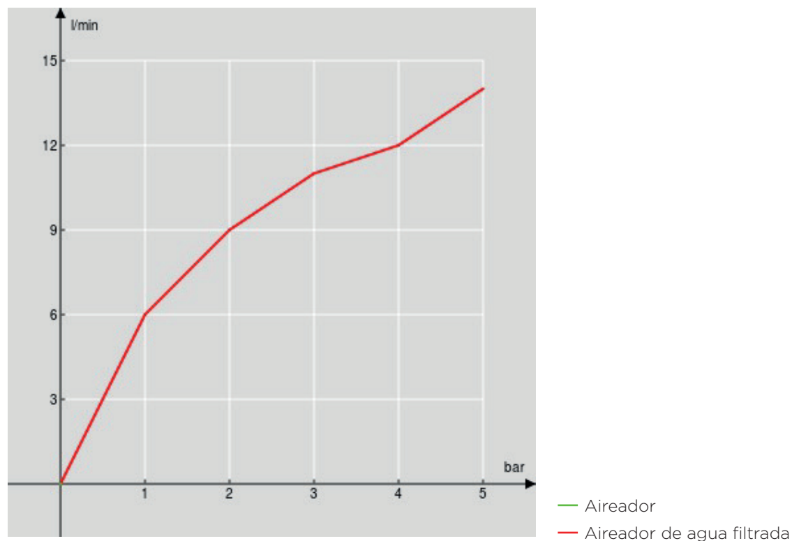
DIAGRAMA DE FLUJO: AGUA MEZCLADA
